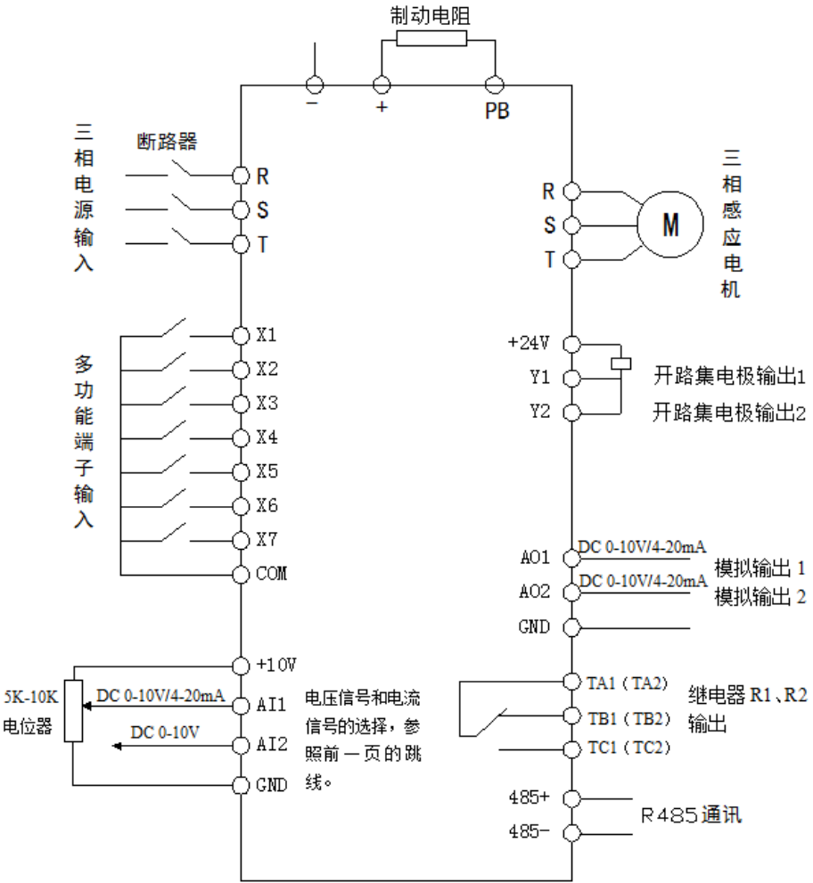
基本运行配线图
